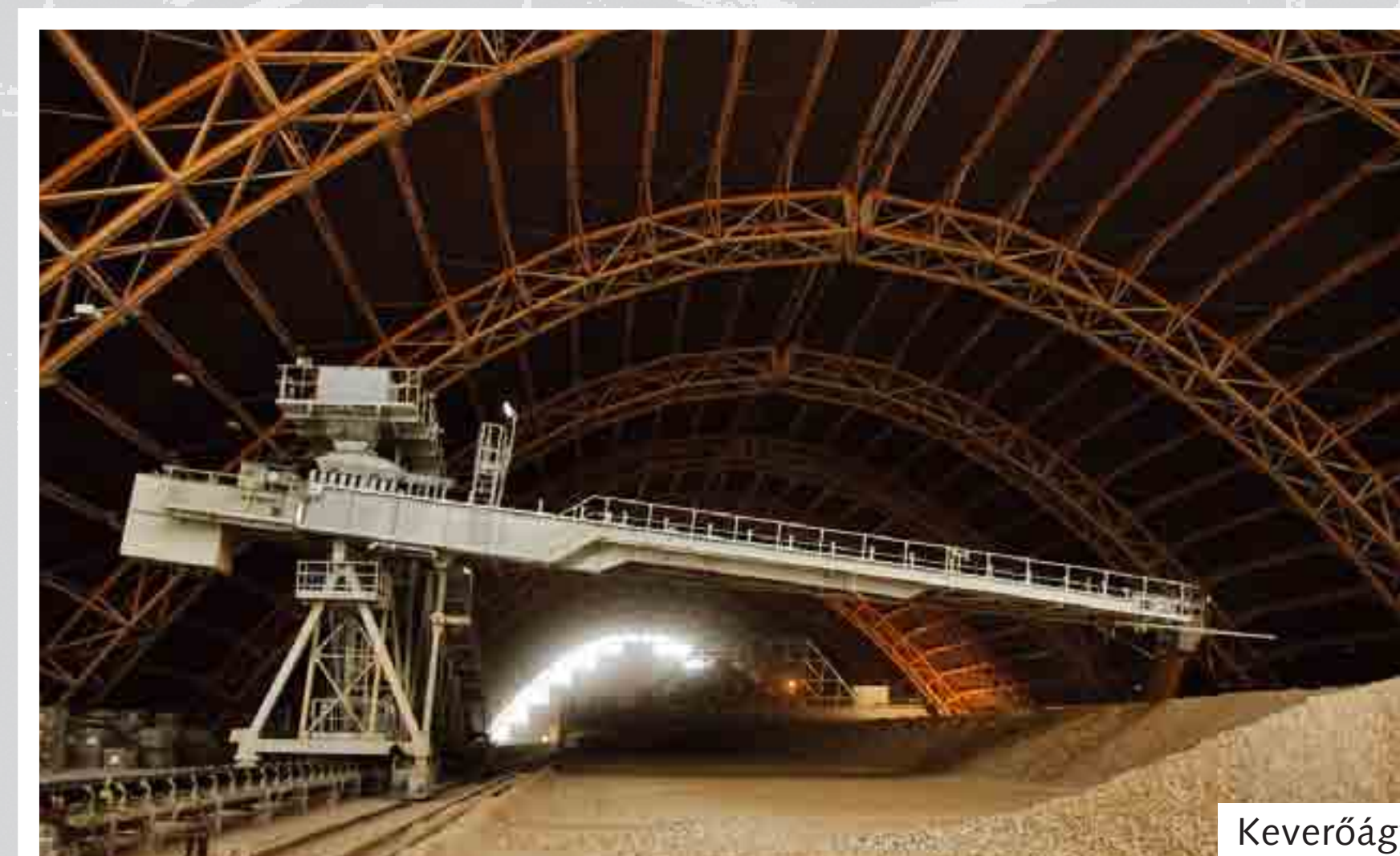
Keverőágy
